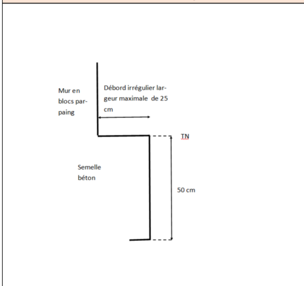
Coupe de la reconnaissance RF4 effectuée
