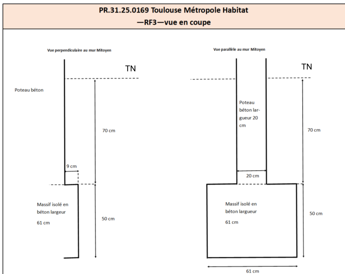
Coupe de la reconnaissance RF3 effectuée
