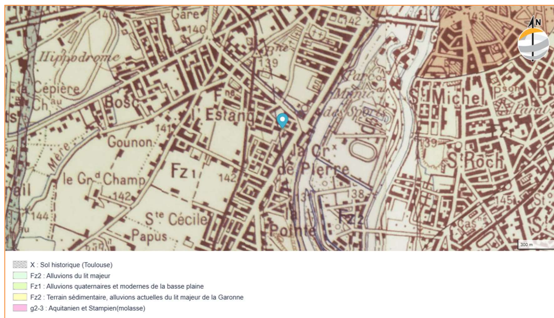
Extrait de la carte géologique de Toulouse Ouest (source : BRGM ©)
